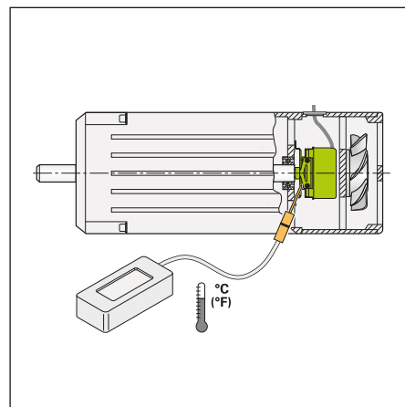
Mesure de la température de service réelle au point de mesure défini sur le capteur rotatif (voir Spécifications techniques )
