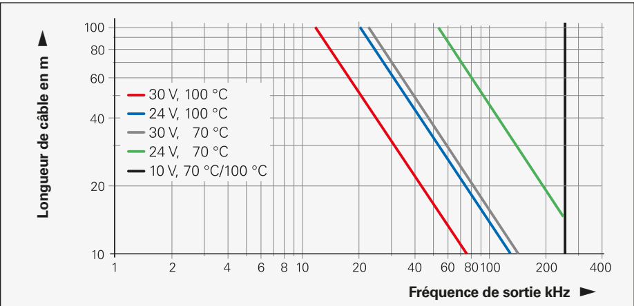
Longueur de câble maximale admissible avec une interface HTLs
