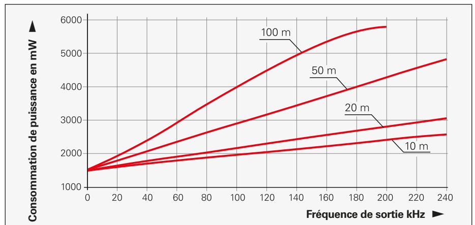
Consommation de puissance (maximale) avec interface HTLs et tension d'alimentation U_P = 30V
