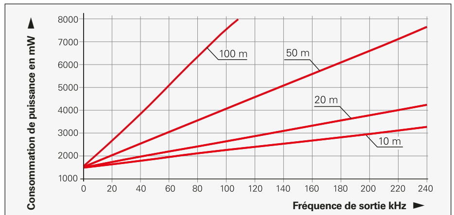
Consommation de puissance (maximale) avec interface HTL et tension d'alimentation U_P = 30V
