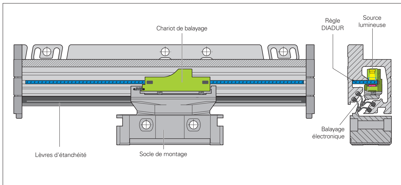
Montage schématisé du système de mesure linéaire étanche LC 115
