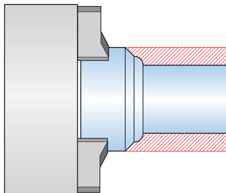
2. Multipasses longitudinales
