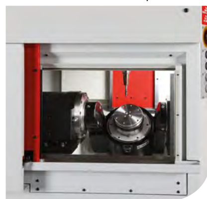
Porta automatica per pallet Automatic door for pallet
